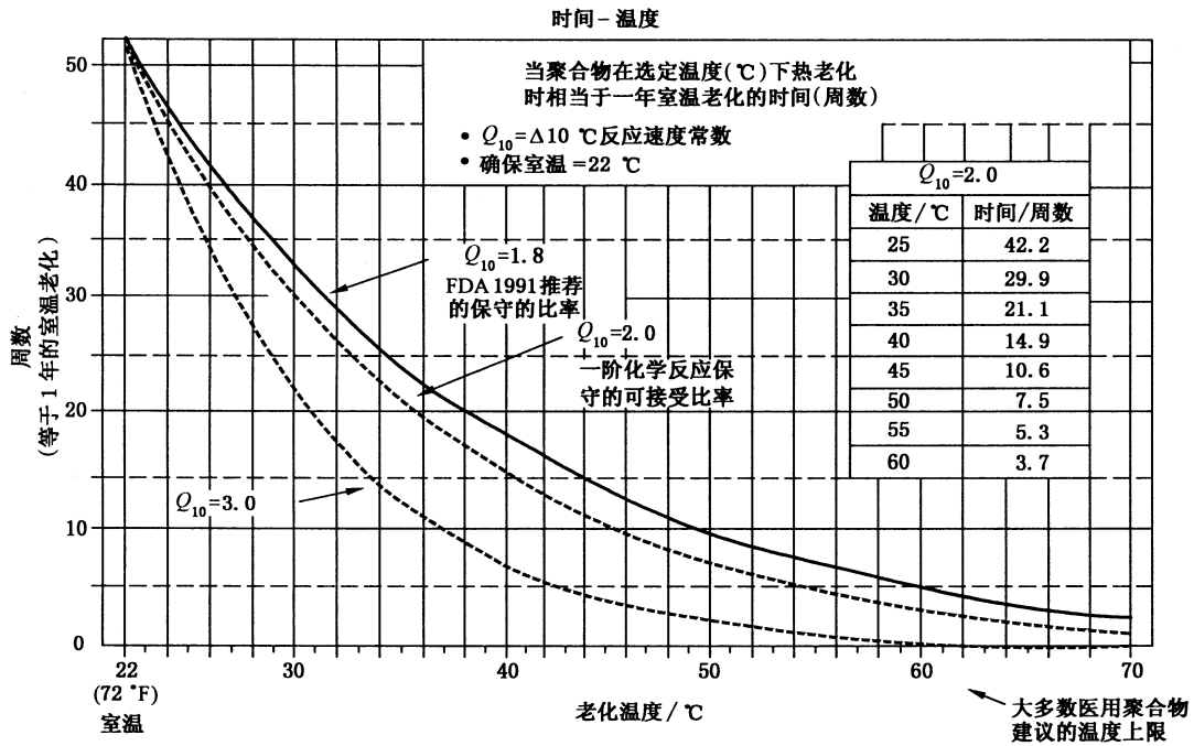
图 A.1 聚合物的加速老化
